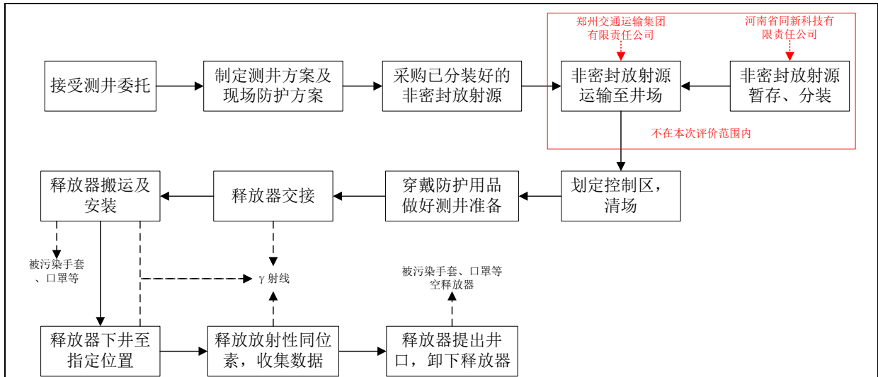
图 9-4 非密封放射源测井工艺流程及产排污环节示意图
