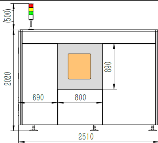
图 10-8 无损检测室（二）铅房立面图
