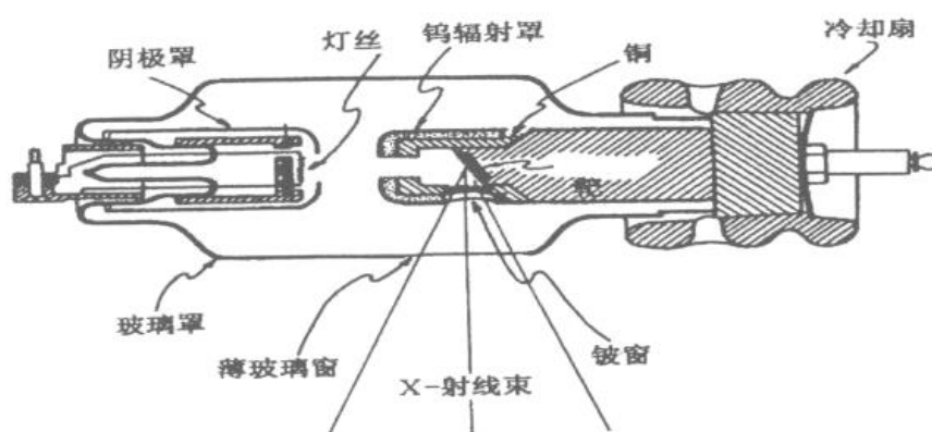
图 9-1 典型的 X 射线管结构图
