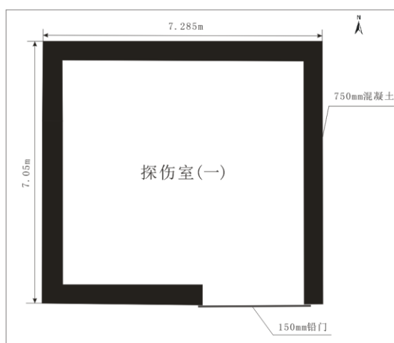
图 10-5 无损检测室（一）平面图
