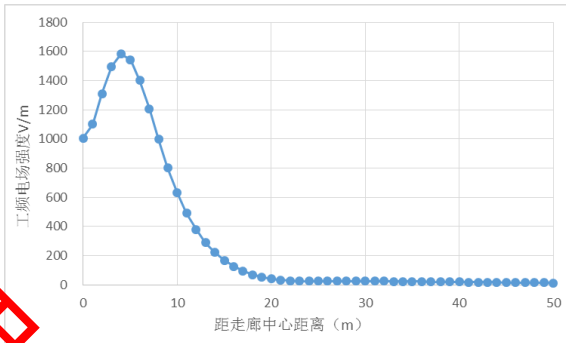
图 10 1D6-SZ2 型塔弧垂高度 7m 工频电场强度随距离变化趋势
