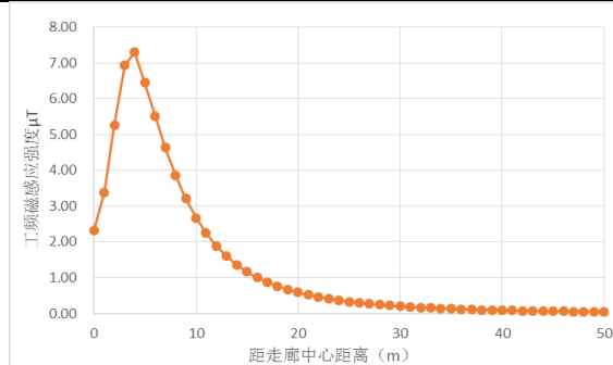
图5 1D6-SZ1型塔弧垂高度6m工频磁感应强度随距离变化趋势
