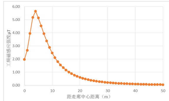
图 11 1D6-SZ2 型塔弧垂高度 7m 工频磁感应强度随距离变化趋势
