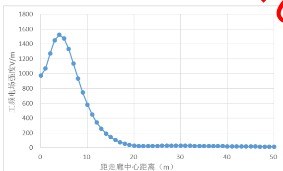
图6 1D6-SZ1型塔弧垂高度7m工频电场强度随距离变化趋势
